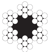
6 x 7 FC
